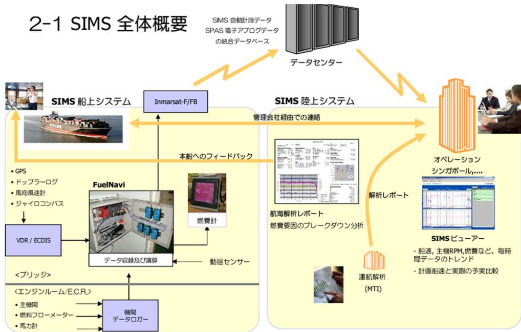
運航モニタリングシステム, SIMS 1)
