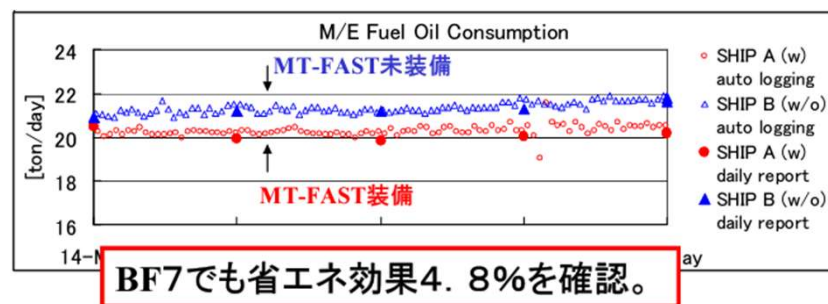
姉妹船の並走試験による省エネ付加物の検証 2)
