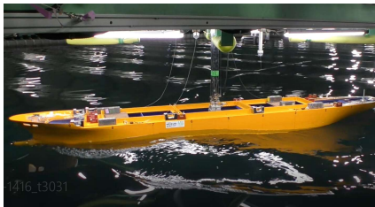
模型(水槽試験)
